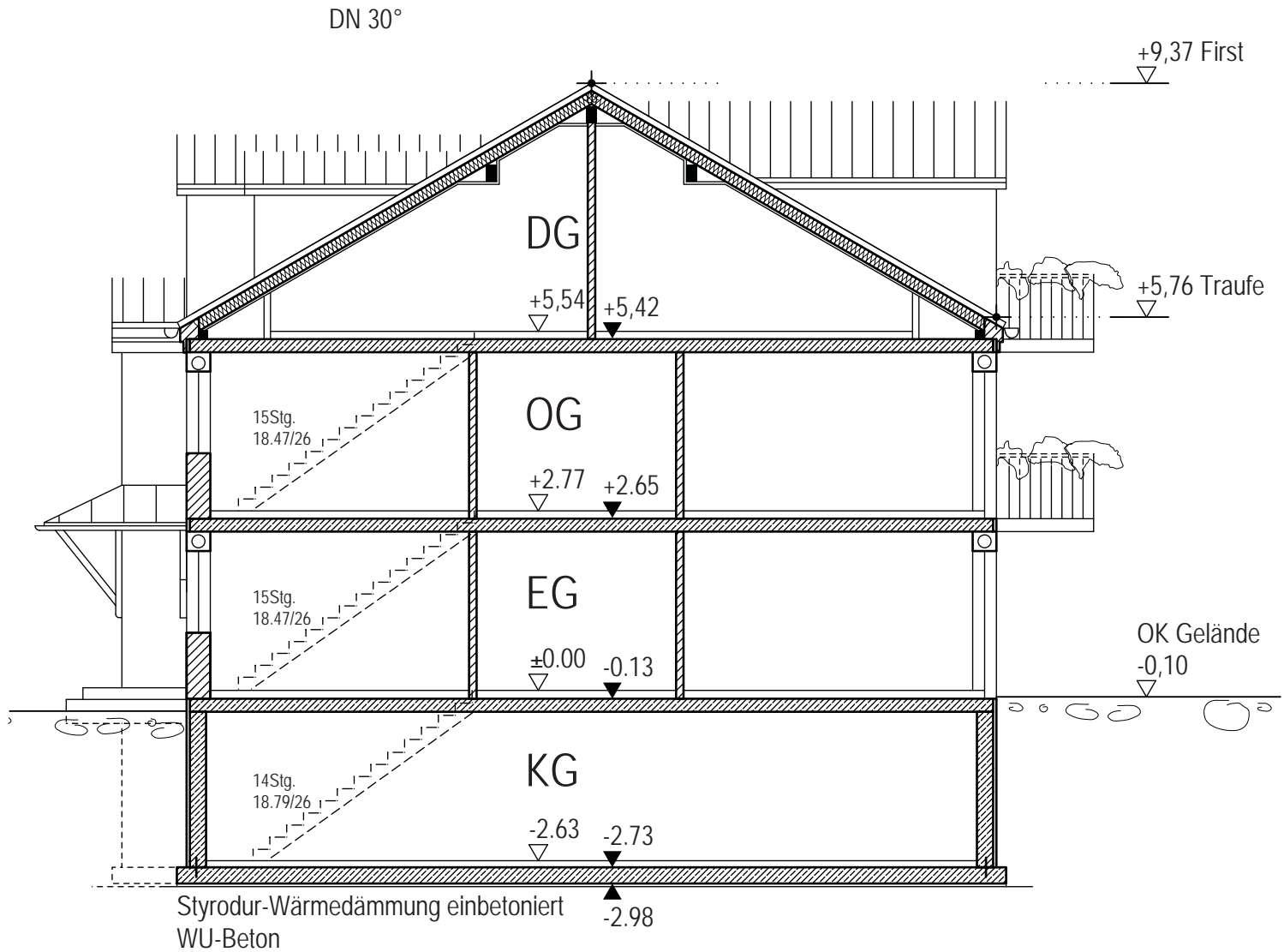
SCHNITT 1-1 HAUS 1+2
