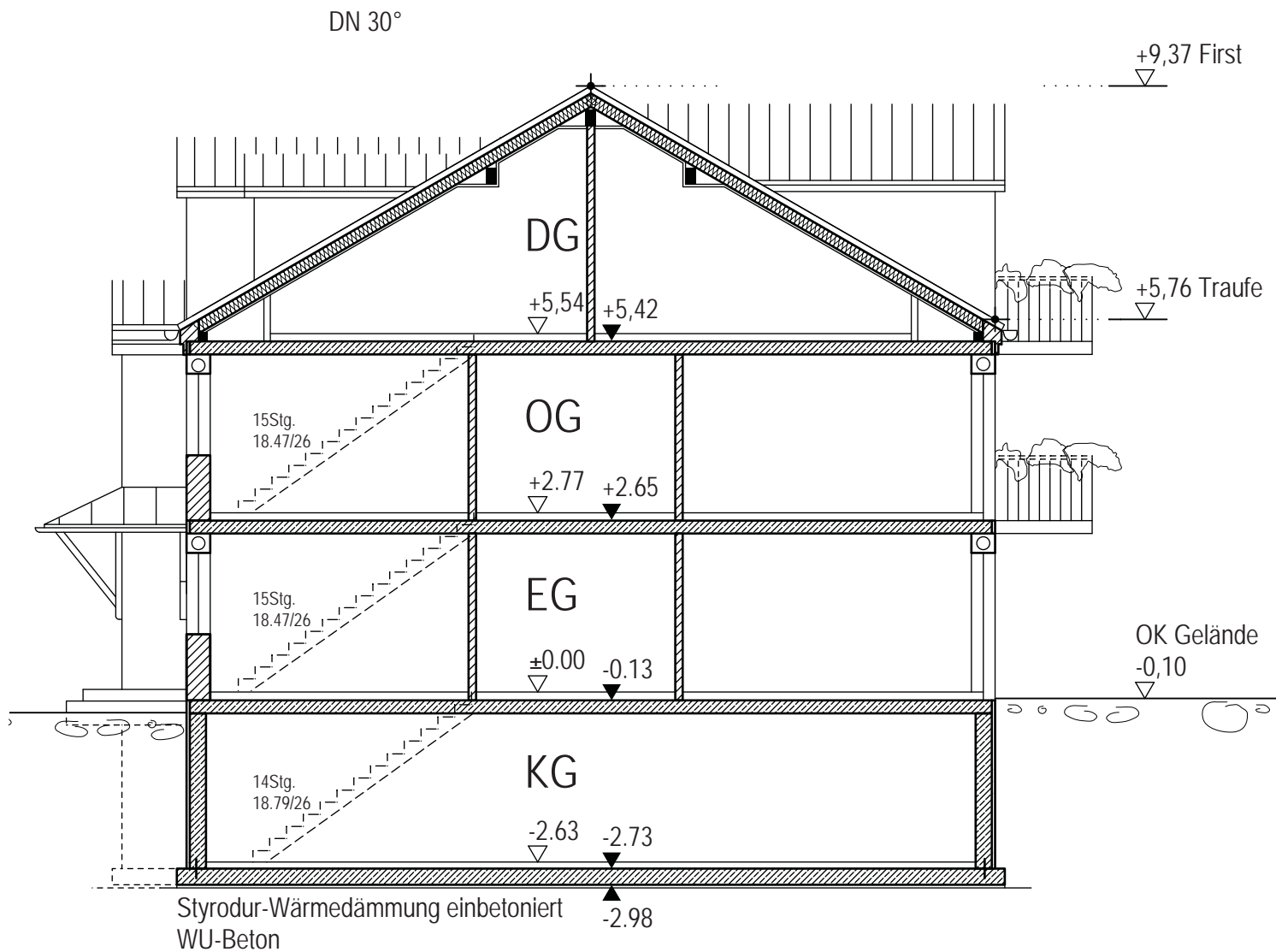
SCHNITT 1-1 HAUS 1+2
