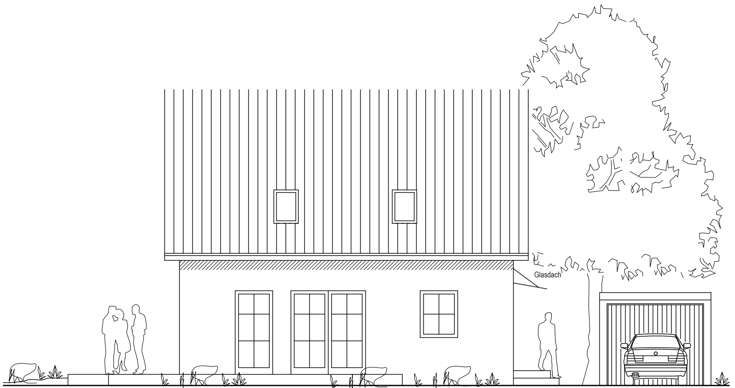
ANSICHT WEST
